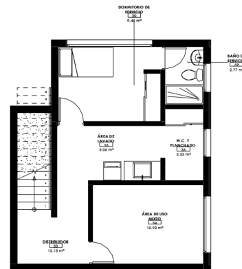
1 PLANTA ARQ. AMUEBLADA SÓTANO 1:50
