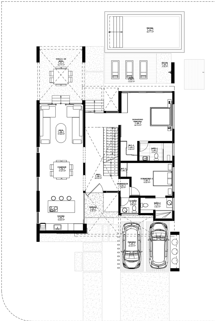
① PLANTA ARQ. AMUEBLADA 1ER NIVEL 1 : 60
