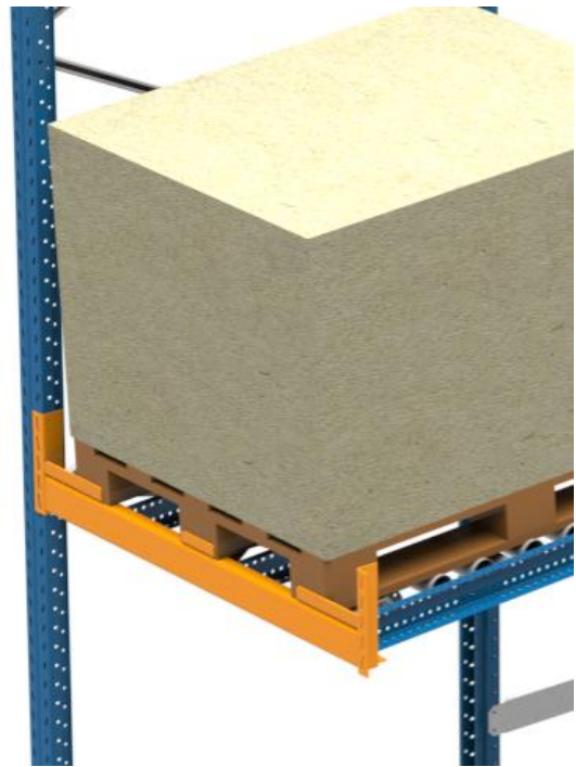
Figura 52 - longarina de saída estrutura dinâmica
