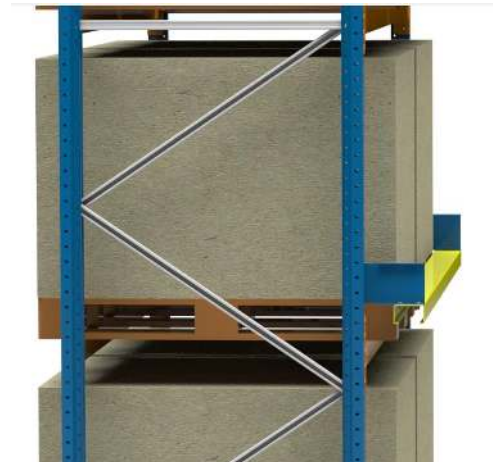
Figura 14 - Vista lateral limitador de fundo
